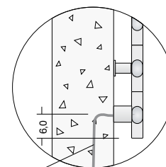
câble d'alimentation de la résistance électrique ou de raccordement du récepteur sans fil à insérer dans une boîte encastrée dans le mur placée au choix à 1,20 cm de l'Add_On
